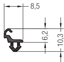
Уплотнение притвора дверной коробки PHZ
