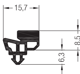
Уплотнение притвора ложного им поста (в комбинации со створками T)
