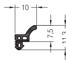
Уплотнение упорной планки шульпы GENEО®
