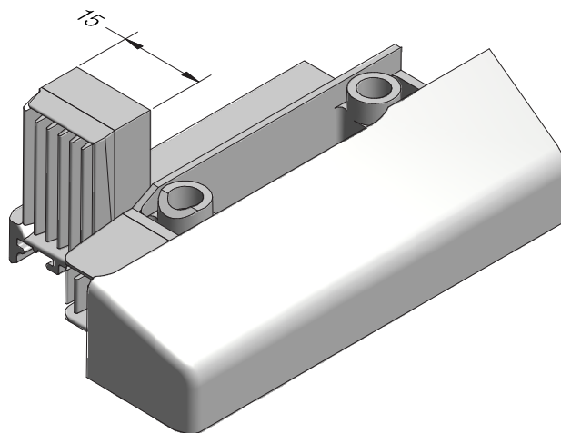
Торцевой колпачок слезника 21 шульп GENEО®
