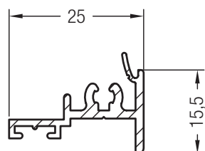
Нащельник створки Т GENEО®
