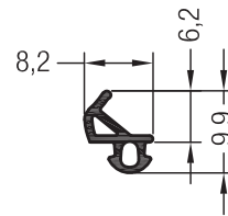
уплотнение притвора EPDM
